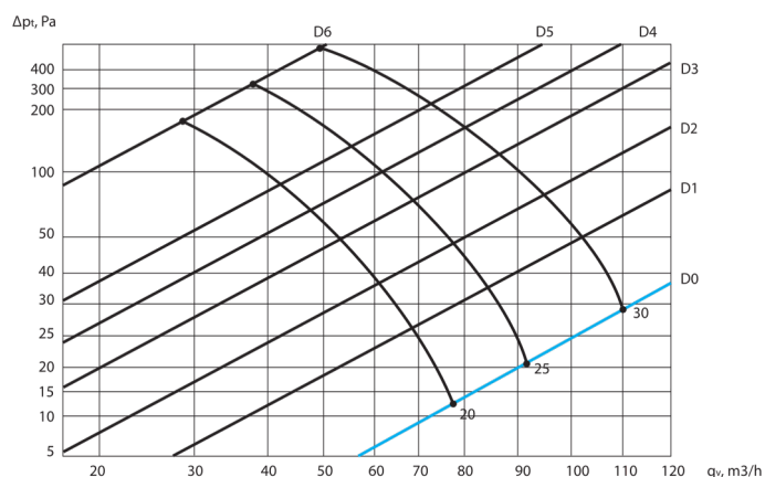
KVADRO 100 (odtah vzduchu)
