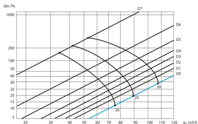
KVADRO 120 (odtah vzduchu)
