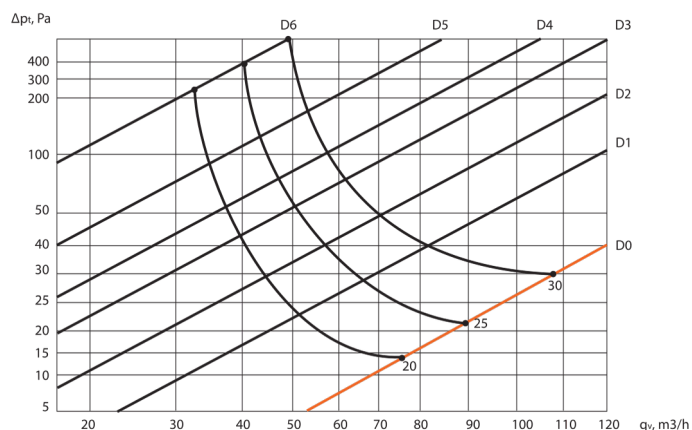
KVADRO 100 (přívod vzduchu)
